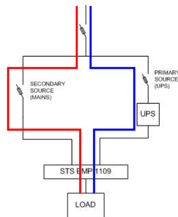
Blok shema ugrađenog STS EMP 1109 Tok energije : plavo – normalan rad;crveno – servis UPS-a
